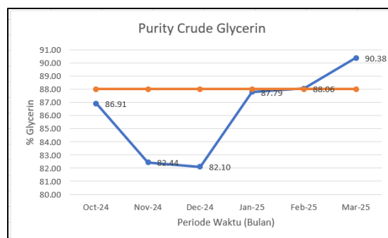
Gambar 3.3 Tren Kualitas Crude Glycerin
