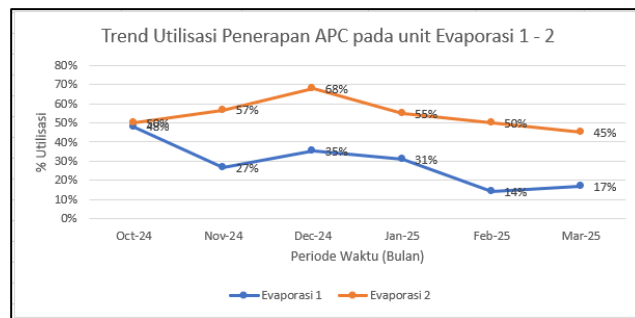
Gambar 3.4 Utilisasi APC Unit Evaporasi 1&2
