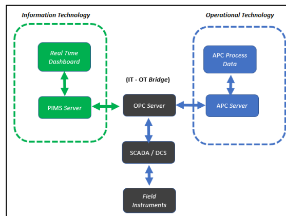
Gambar 3.9 Skema Integrasi Aplikasi APC dan PIMS
